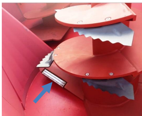
Магнит на витке шнека
